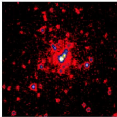
Rosat
