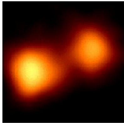
Rosat
